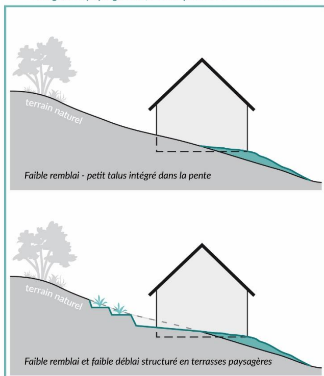
Intégration paysagère et faible impact sur le terrain naturel
