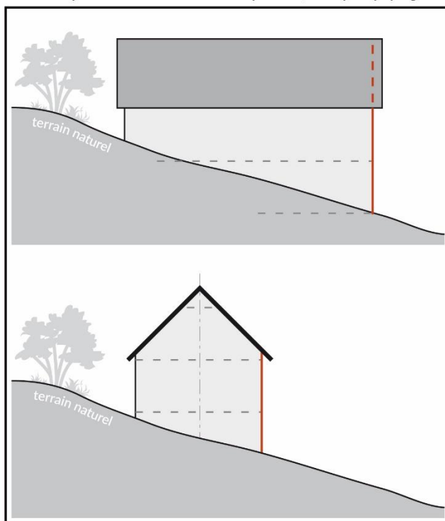
Exemples de constructions dans la pente à fort impact paysager
